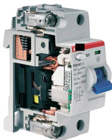
Рисунок 4. Пример конструкции УДТ
